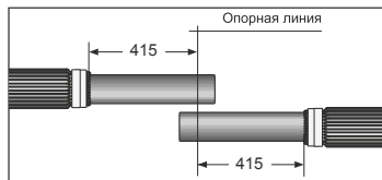
Симметричная разделка кабеля
