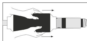
Сборка муфты выполняется без использования инструмента
