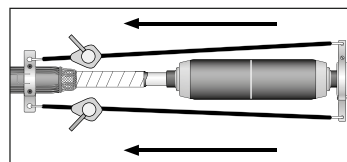
Предварительная парковка стресс-конуса (требуется специальный инструмент)
