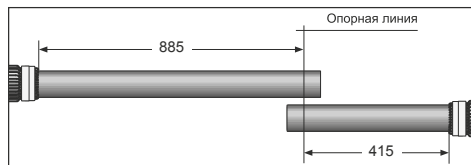
Несимметричная разделка кабеля
